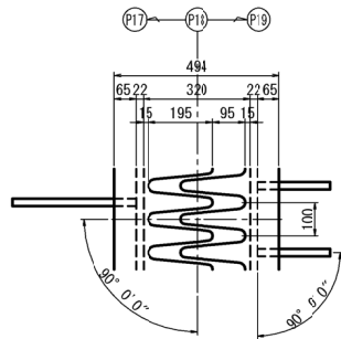
フェイスプレート詳細図 S=1:25
