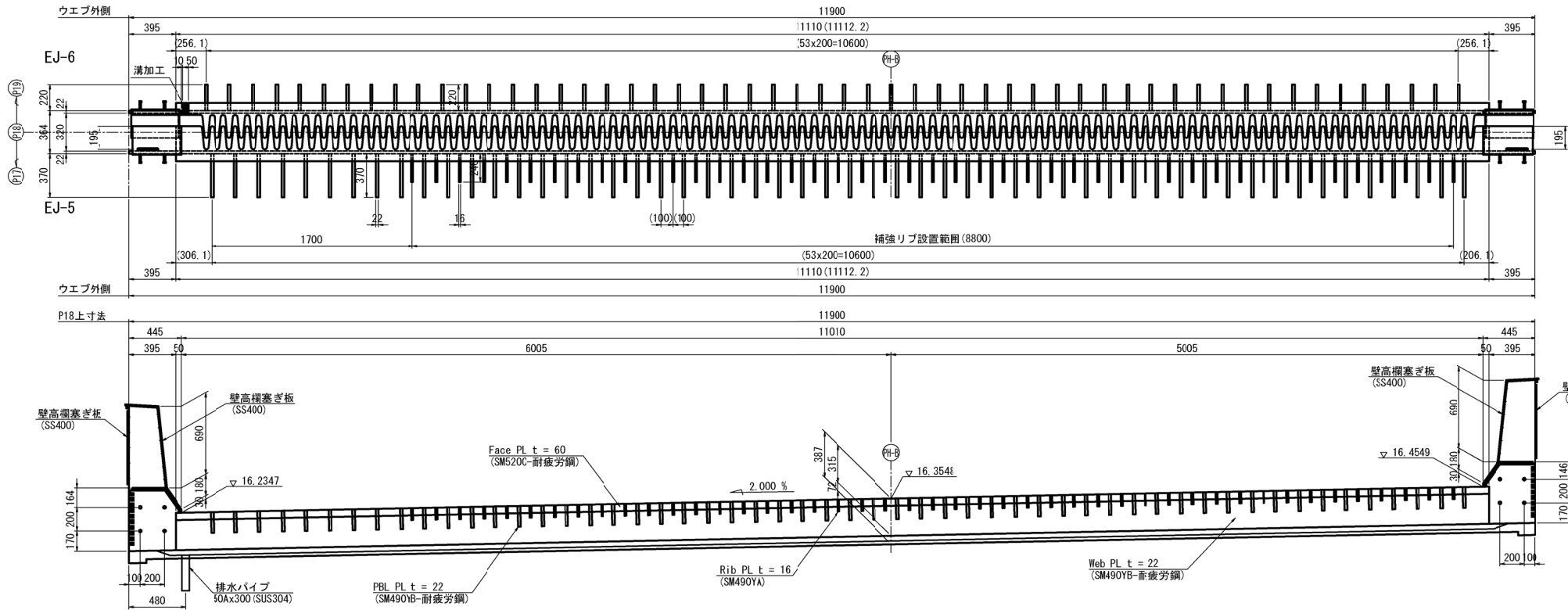
壁高欄塞ぎ板詳細図 S=1:25
