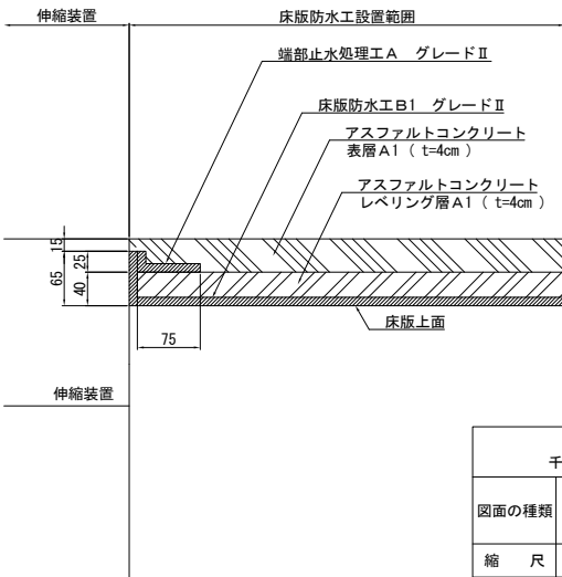
橋軸方向断面図（伸縮装置部） S=1:10
