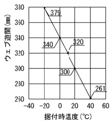
遊間グラフ
