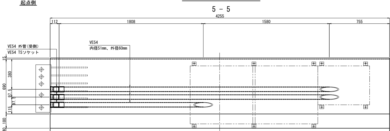
埋設管配置側面図
