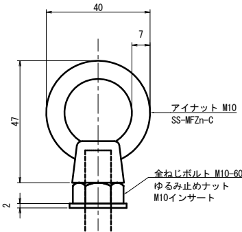
アイナット部詳細図 S=1:2
