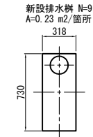
排水柵平面図 S=1:50
