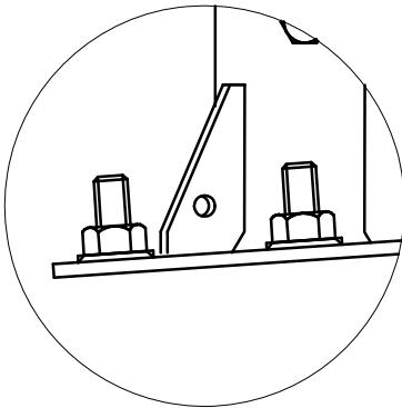
ワイヤー用穴部 S=1:2
