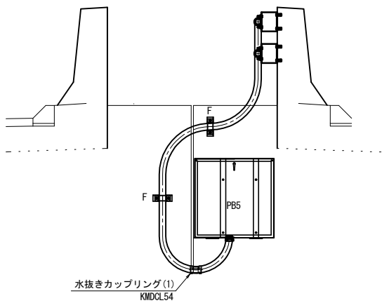
A1橋台正面図
