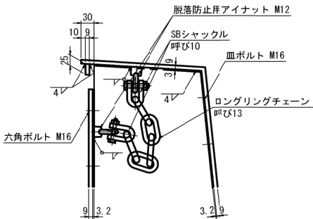
“a”部詳細図 S=1:12.5
