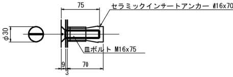
取付ボルト詳細 S=1:7.5
