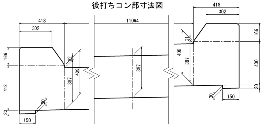
後打ちコン部寸法図
