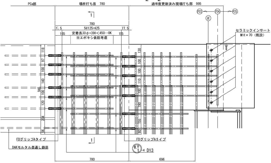
側面図
