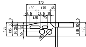
補強リブ詳細図 S=1:25
