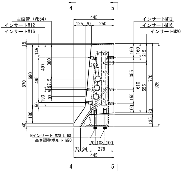
断面図
