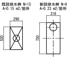
排水樹平面図 S=1:50
