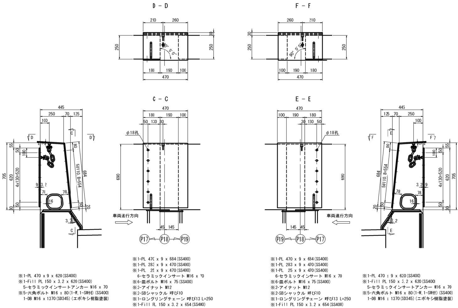
壁高欄塞ぎ板詳細図
