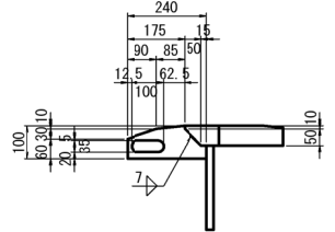
補強リブ詳細図 S=1:25
