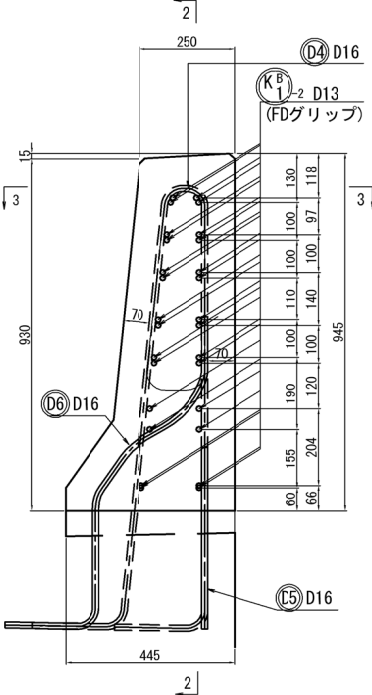
断面図
