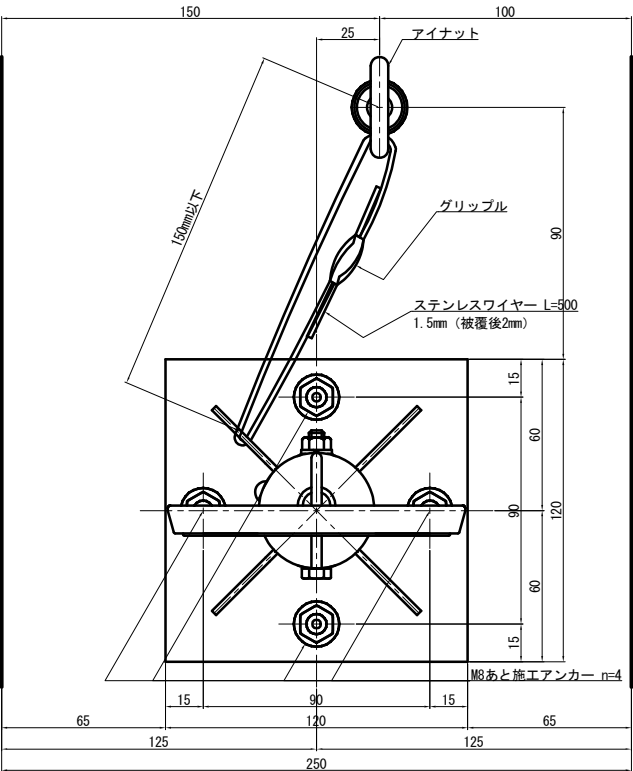
上面図 S=1:3
