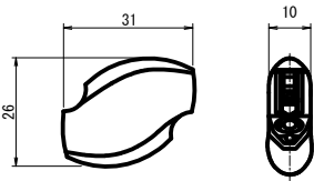
グリップル詳細図 S=1:2
