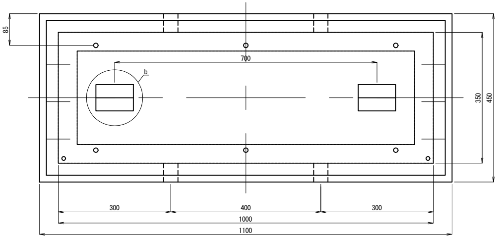
正面図
