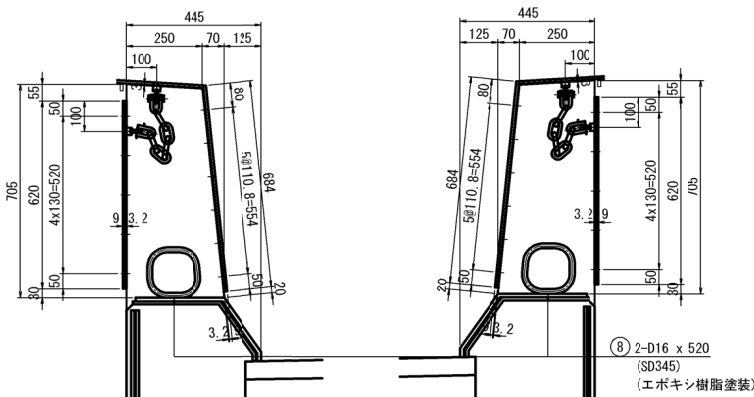
壁高欄塞ぎ板詳細図 S=1:25
