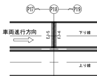
配置図
