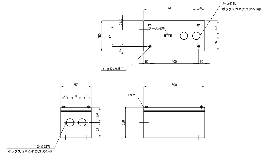
プルボックス
