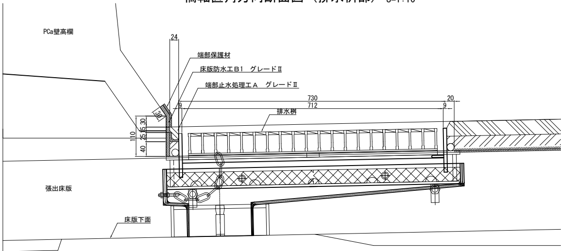
橋軸直角方向断面図（排水柵部） S=1:10
