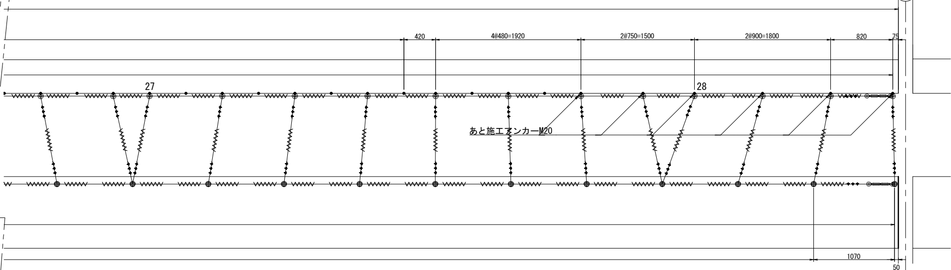
側面図 S=1:50
