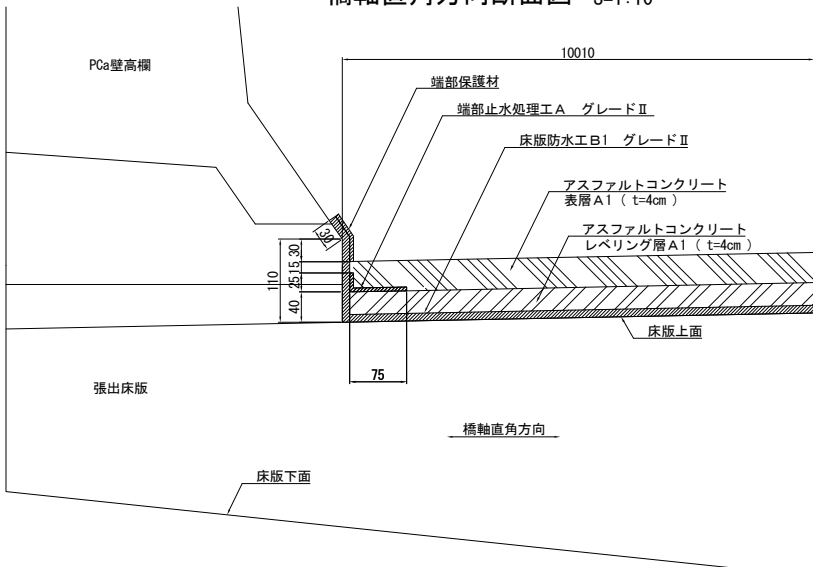
橋軸直角方向断面図 S=1:10
