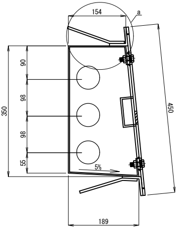
断面図
