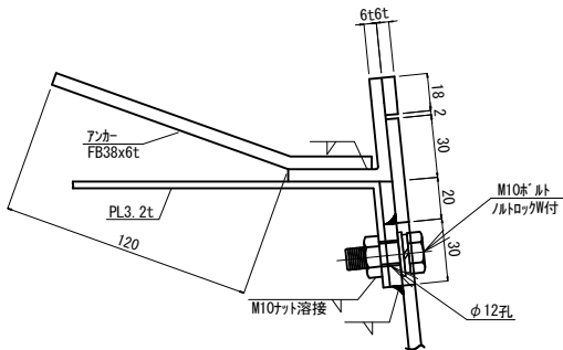
a部詳細図 S=1:4
