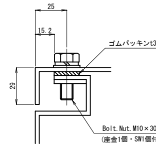
蓋部詳細図
