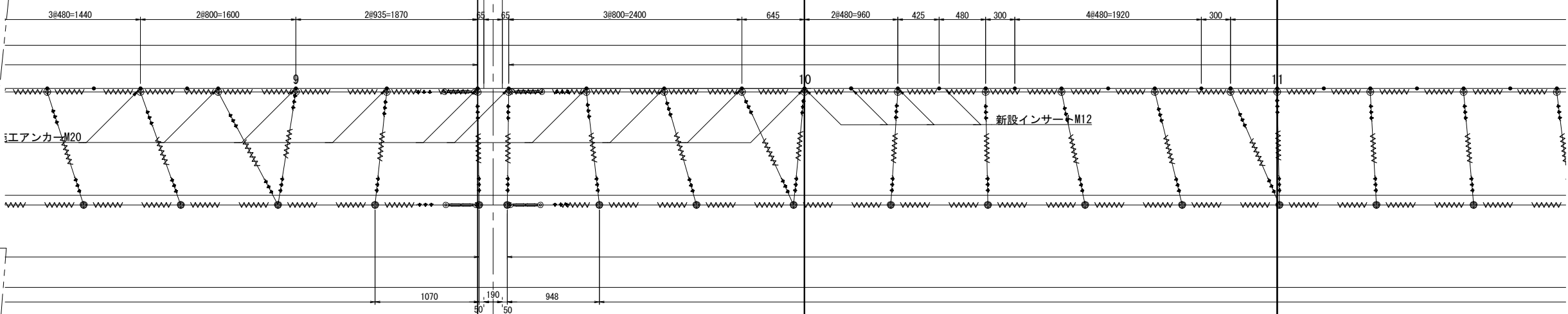
側面図 S=1:50
