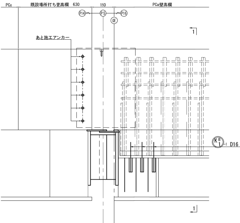
側面図
