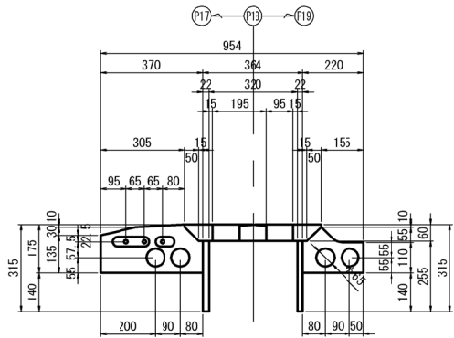
フェイスプレート詳細図 S=1:25
