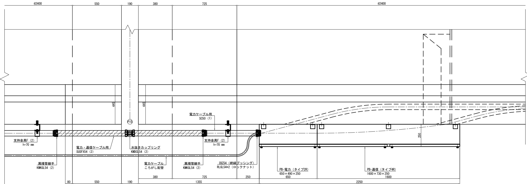
平面図
