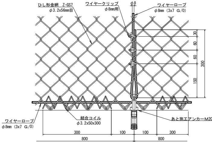
金網およびワイヤーロープ取付詳細図 S=1:10
